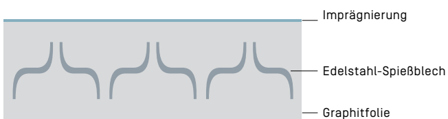
↑ Lagenaufbau
