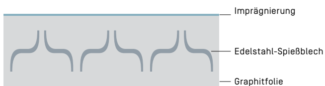
↑ Lagenaufbau
